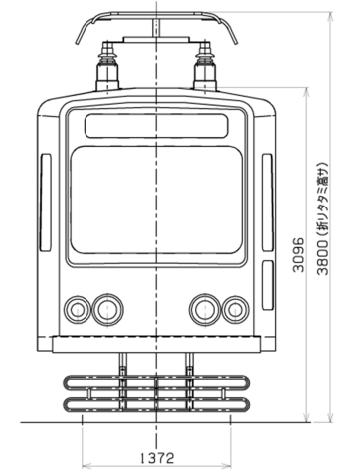
東京都交通局車両電気部車両課 7700形 車両形式図
