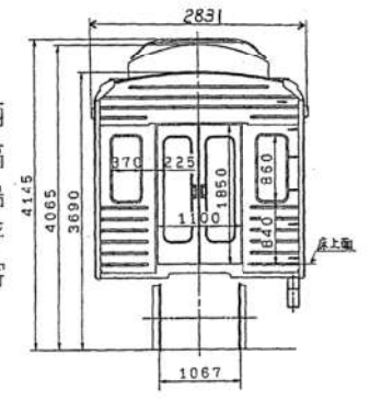
視A-A
