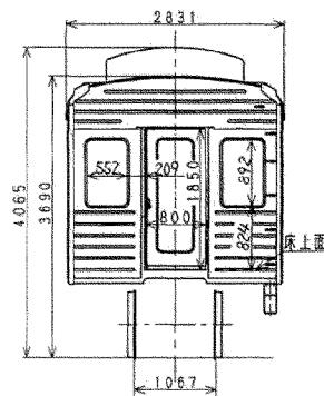
視A-A
