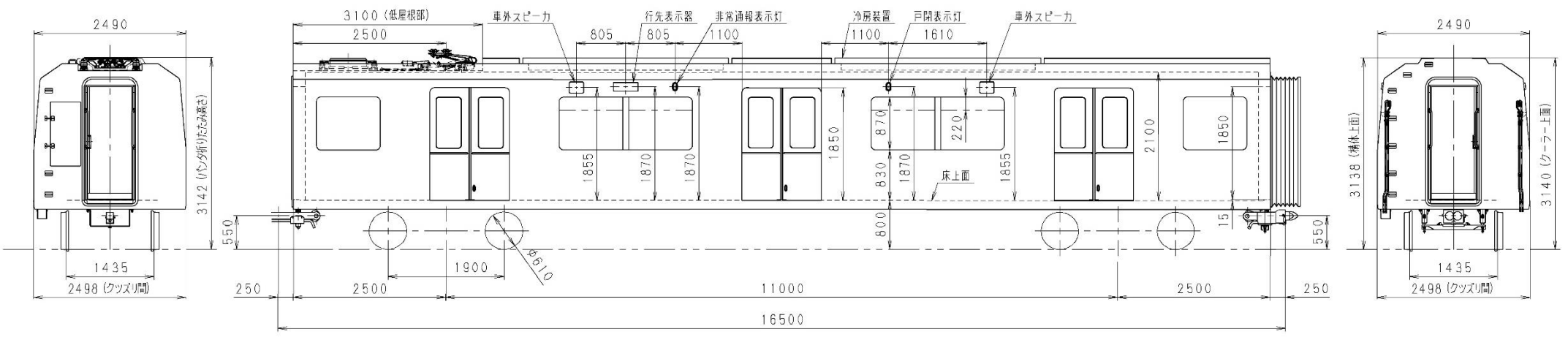
東京都交通局車両電気部車両課 12-600形3,4次車(4号車)車両形式図
