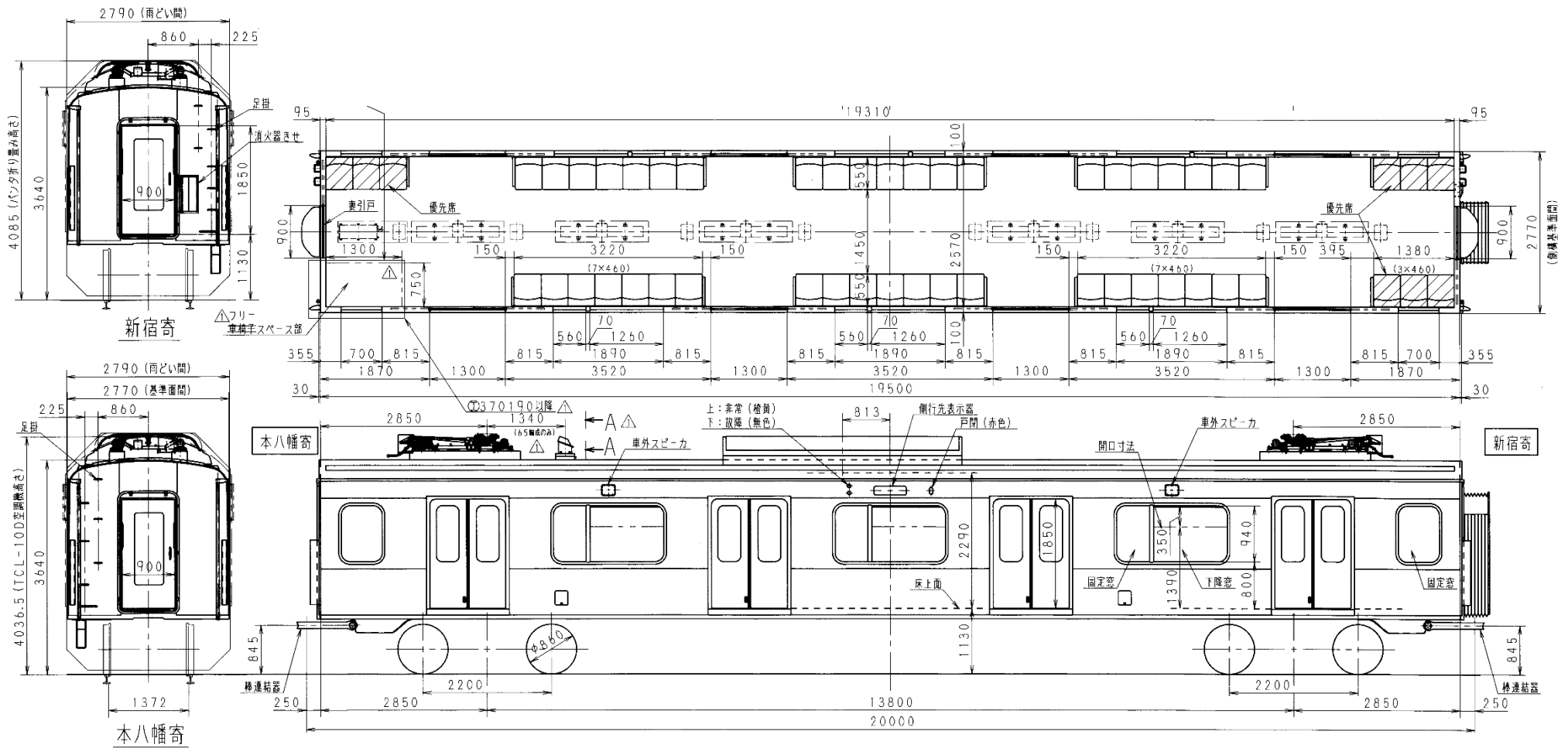
東京都交通局車両電気部車両課 10-300形5.6次車(1号車)車両形式図 フリースペース車
