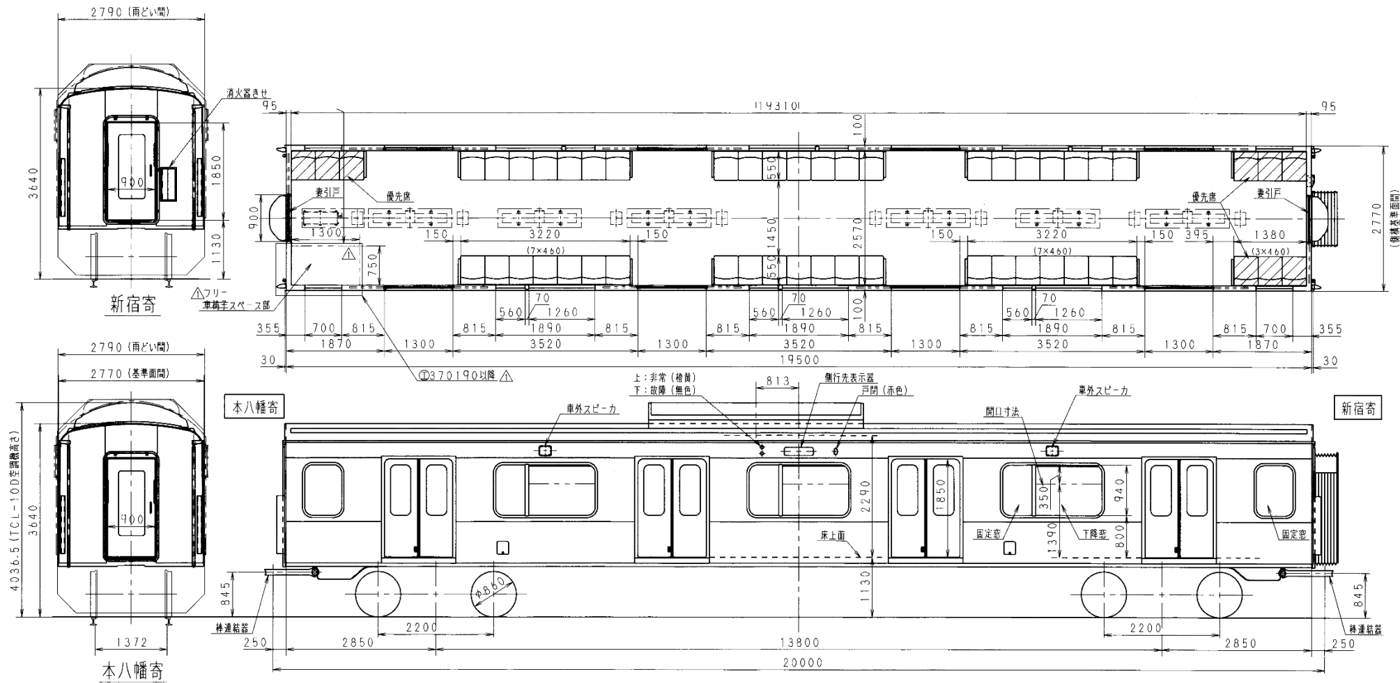
東京都交通局車両電気部車両課 10-300形5.6次車(8号車)車両形式図 フリースペース車
