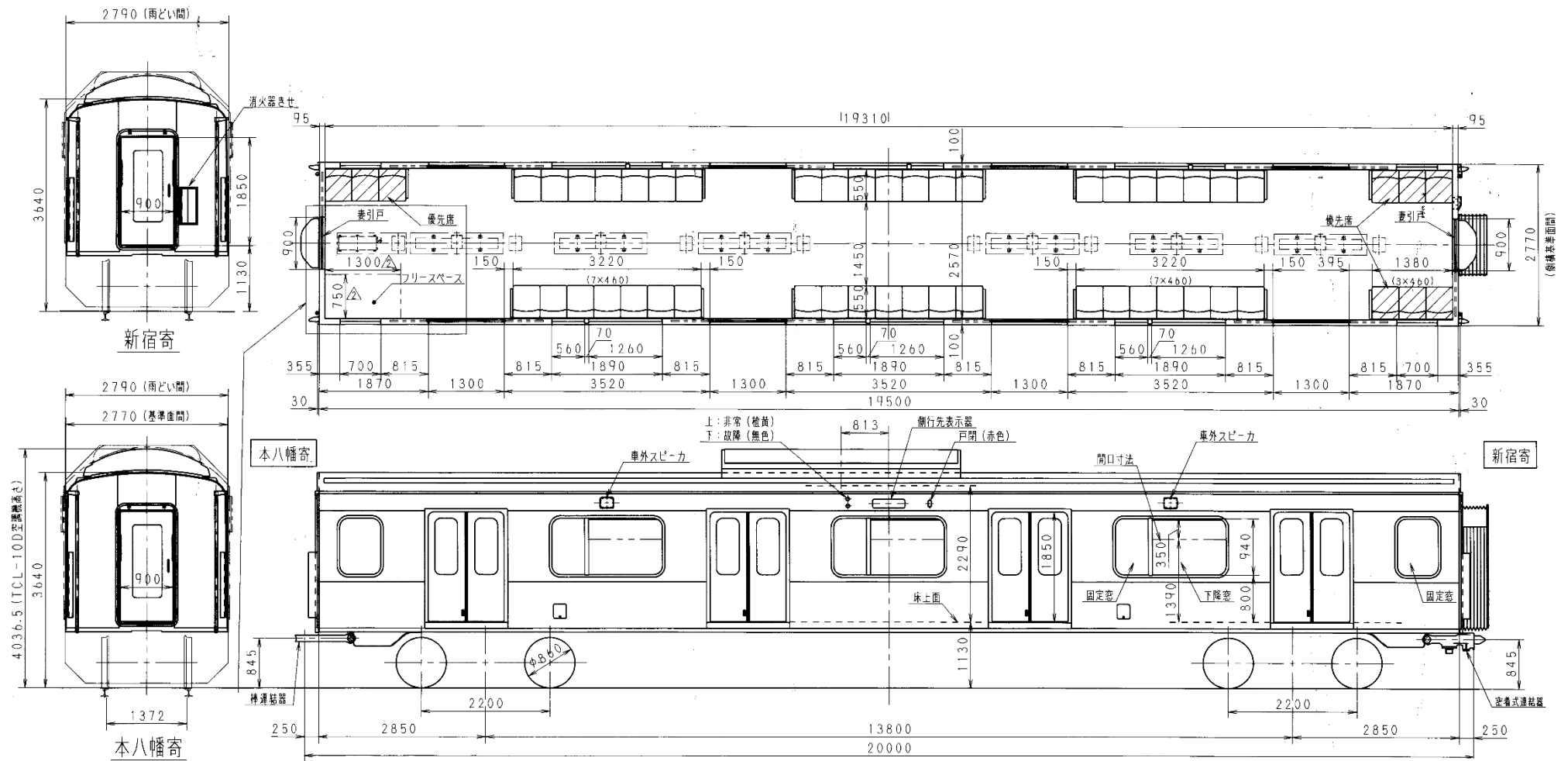
東京都交通局車両電気部車両課 10-300形5.6次車(2.4号車)車両形式図 フリースペース車
