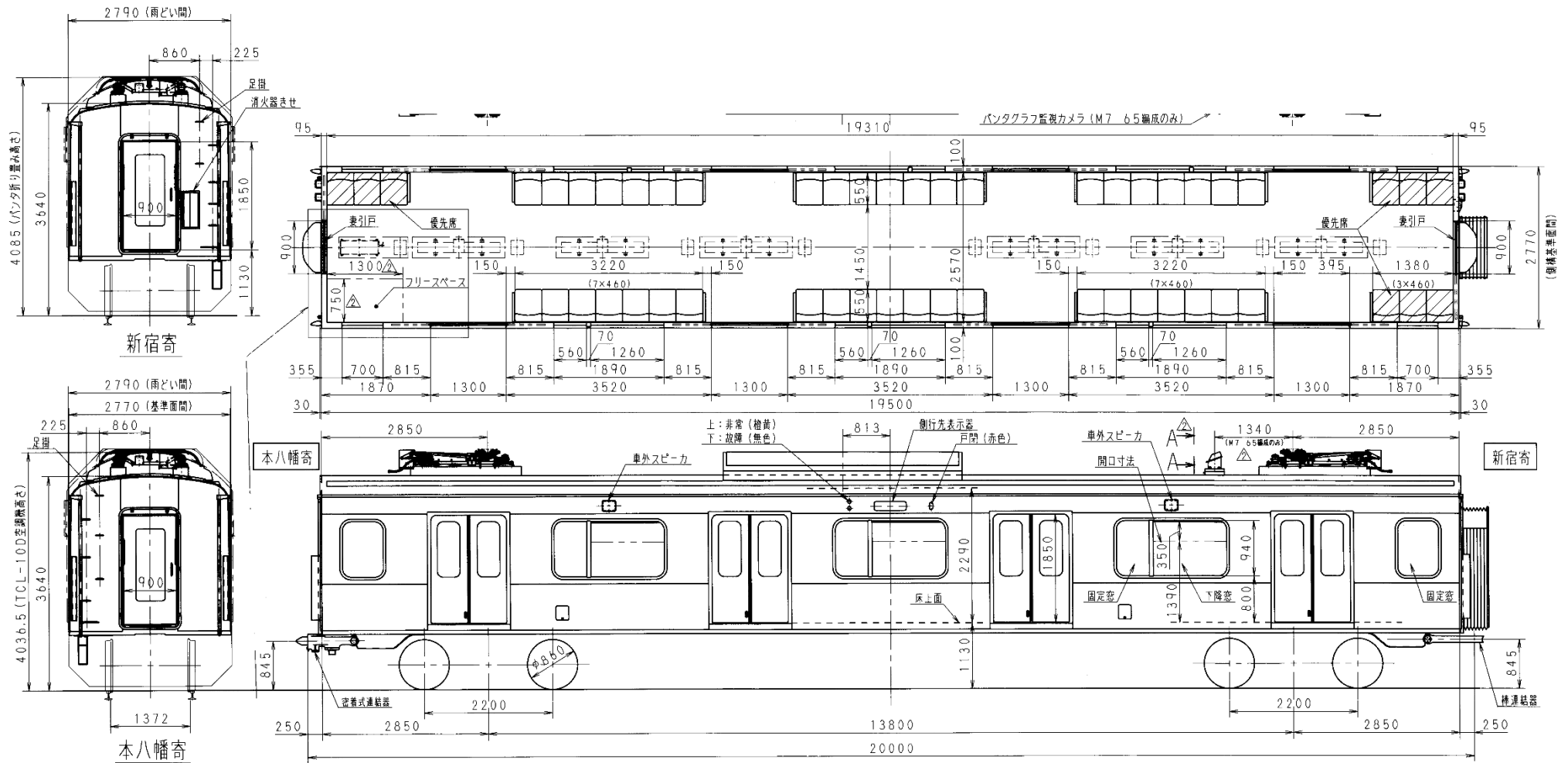
東京都交通局車両電気部車両課 10-300形5.6次車(3.7号車)車両形式図 フリースペース車
