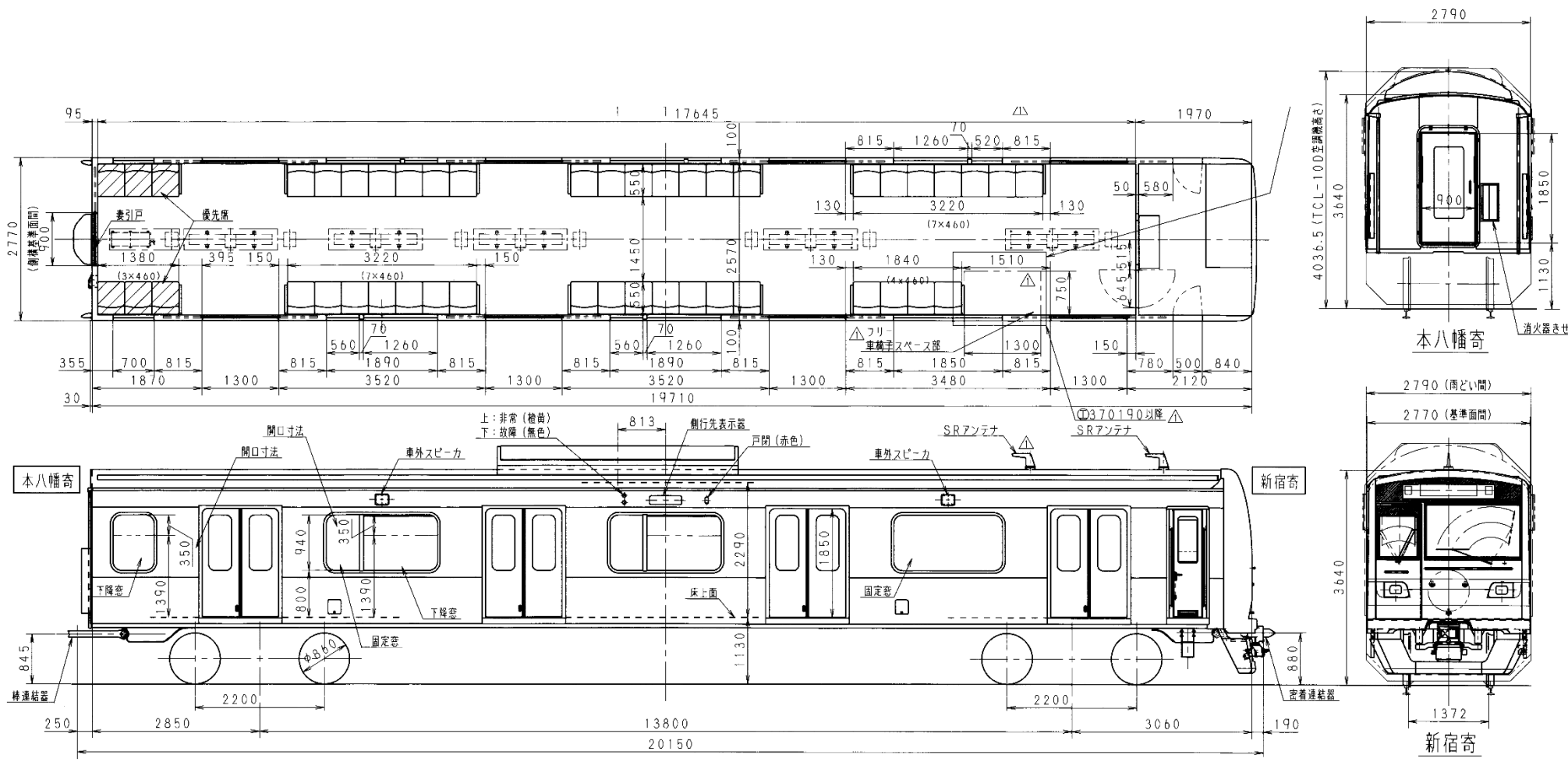
東京都交通局車両電気部車両課 10-300形5.6次車(9号車)車両形式図 フリースペース車
